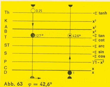
Abb. 63 \varphi = 42,6^\circ
