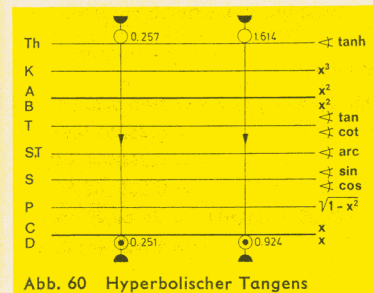
Abb. 60 Hyperbolischer Tangens
