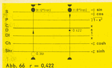
Abb. 66 r = 0,422
