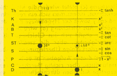
Abb. 69 \varphi = 4,68^\circ
