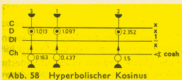
Abb. 58 Hyperbolischer Cosinus
