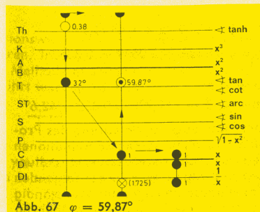
Abb. 67 \varphi = 59,87^\circ
