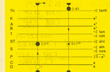
Abb. 77 r = 0,976
