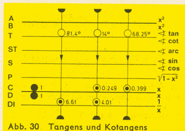
Abb. 30 Tangens und Kotangens
