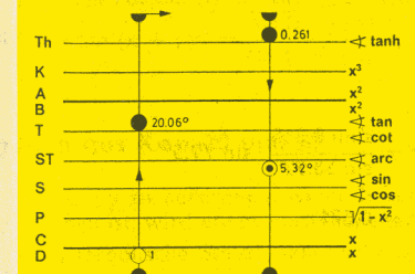
Abb. 75 r = 0,954
