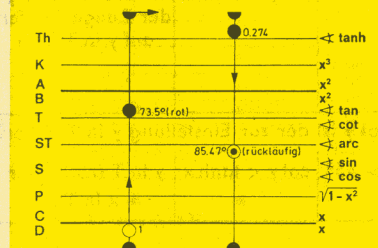
Abb. 71 \varphi = 85,47^\circ
