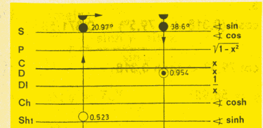
Abb. 75 r = 0,954
