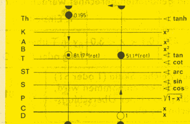
Abb. 70 \varphi = 81,17^\circ
