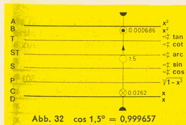
Abb. 32 \cos 1,5^\circ = 0,999657
