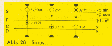
Abb. 28 Sinus
