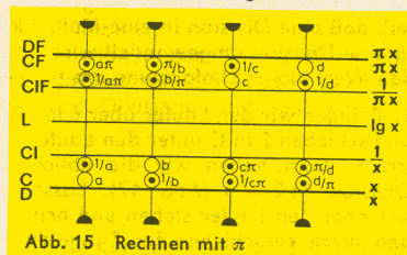
Abb. 15 Rechnen mit \pi
