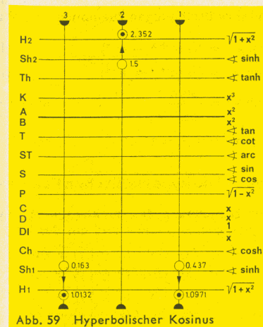
Abb. 59 Hyperbolischer Kosinus
