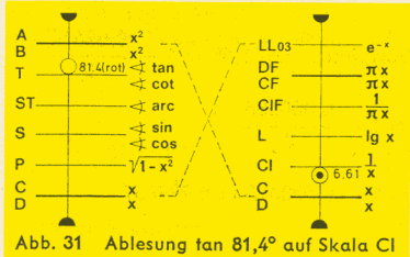
Abb. 31 Ablesung \tan 81,4^\circ auf Skala CI
