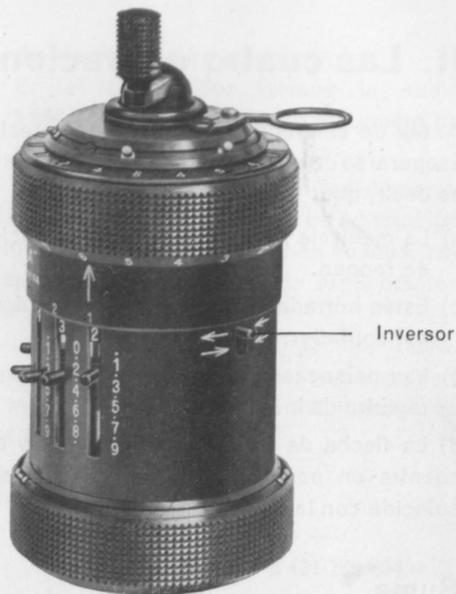
Fig. 8. La Curta vista por detrás
