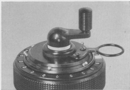
Fig. 5. La manivela sacada en posición de resta
